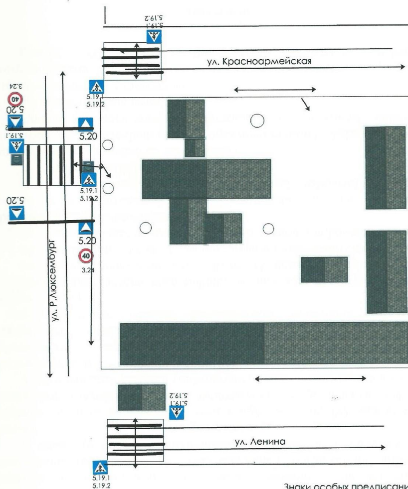
2. Схема организации дорожного движения в непосредственной близости от гимназии с размещением существующих технических средств организации дорожного движения, маршрутов движения детей и расположения парковочных мест
